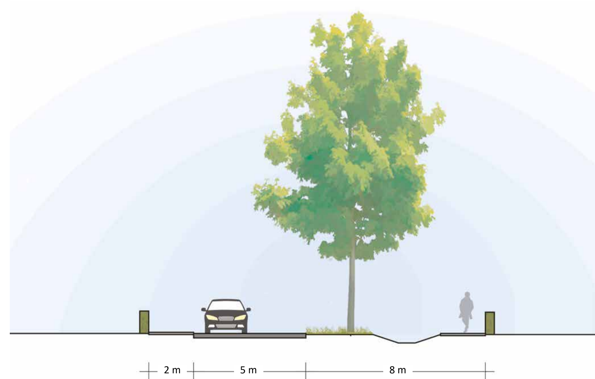
Profiel 6: ontsluitingsweg zuidzijde
