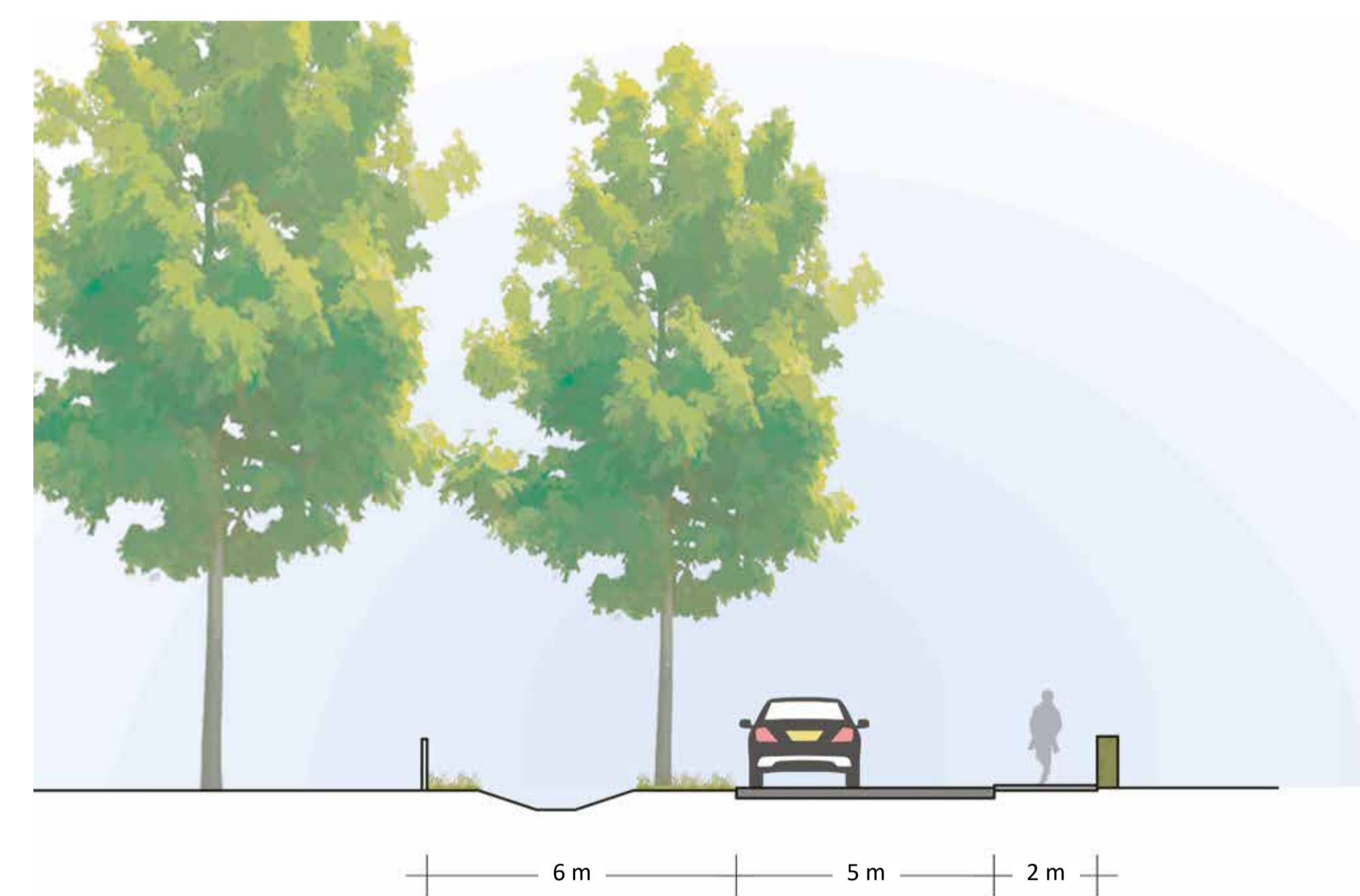
Profiel 8: toegangsweg Heiligenboom
